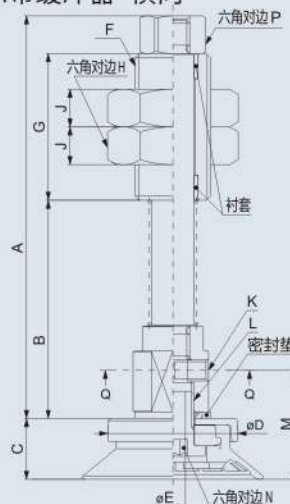
UM带缓冲器-横向
