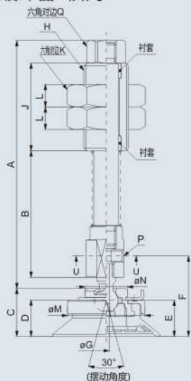
UM带缓冲器-横向
