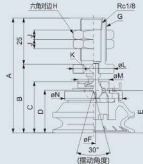
BM外螺纹安装-纵向
