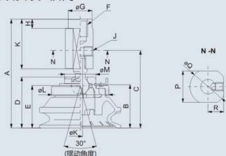
BM内螺纹安装-横向
