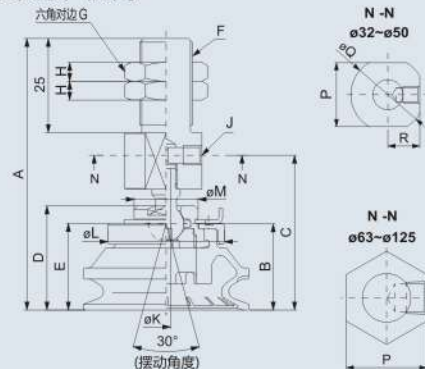
BM外螺纹安装-横向
