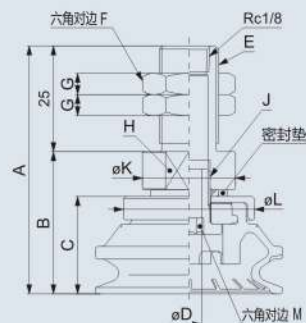
BM外螺纹安装-纵向
