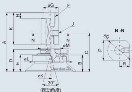
UM内螺纹安装-横向
