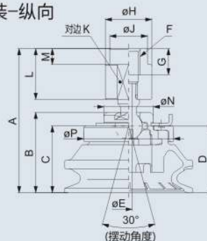
BM内螺纹安装-纵向
