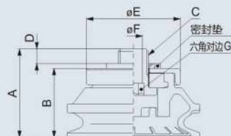
BM带锁定螺钉-纵向
