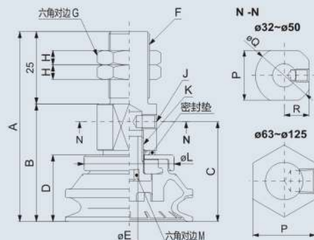
BM外螺纹安装-横向
