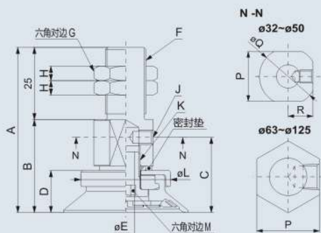
UM外螺纹安装-横向
