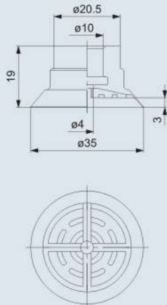
ZP3P-35PTSF 净重：5.8g
