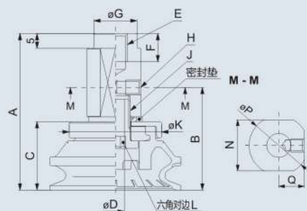
BM内螺纹安装-横向
