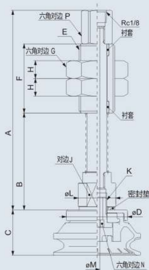
BM带缓冲器-纵向
