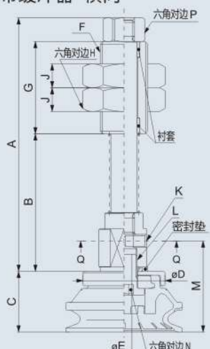
BM带缓冲器-横向
