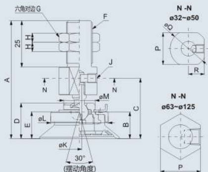
UM外螺纹安装-横向
