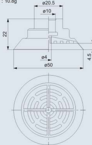
ZP3P-50PTSF 净重：10.8g
