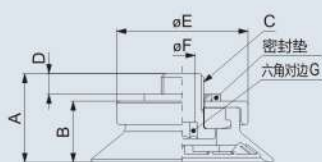
UM带锁定螺钉-纵向
