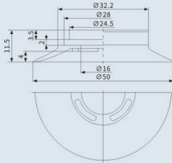
适合吸盘直径 Ø50
