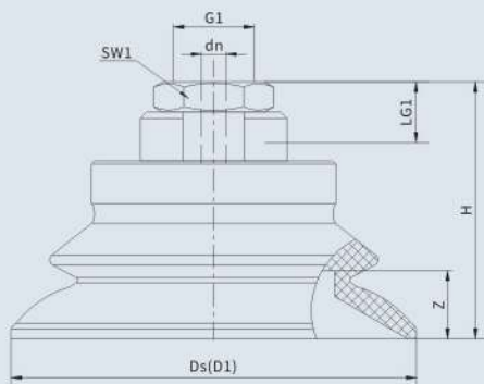
•MAB30~100IG(内螺纹)
