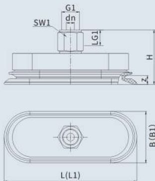
•MAOB60x30~110x55 (内螺纹)
