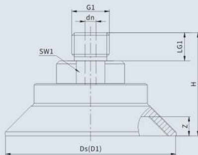
•MAF30~100AG(外螺纹)
