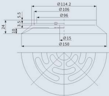
适合吸盘直径 Ø150
