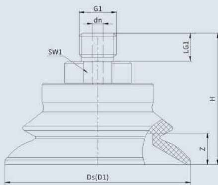
•MAB30~100AG(外螺纹)
