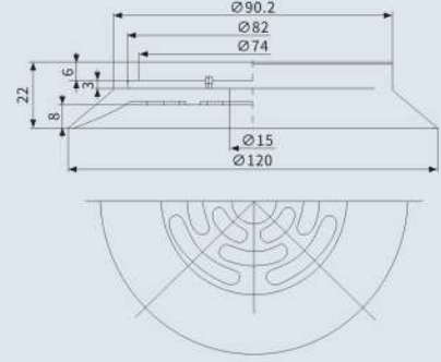
适合吸盘直径 Ø120
