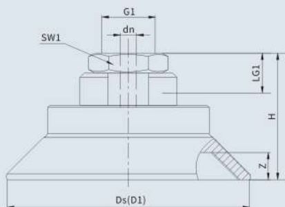
•MAF30~100IG(内螺纹)
