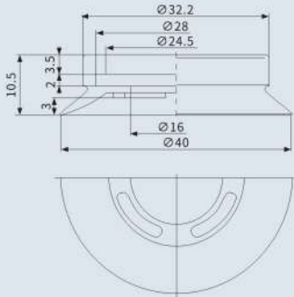
适合吸盘直径 Ø40
