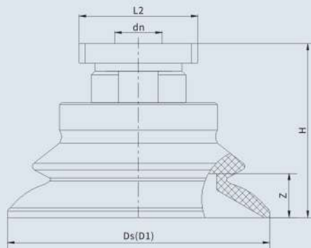
•MAB30~100RA(矩形适配器)
