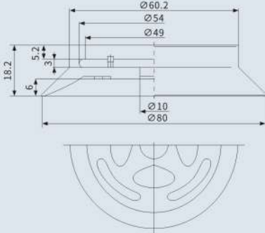
适合吸盘直径 Ø80
