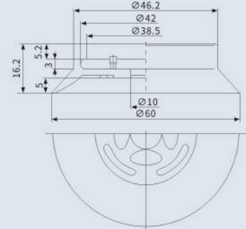
适合吸盘直径 Ø60
