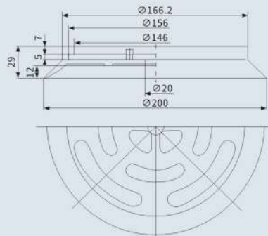
适合吸盘直径 Ø200
