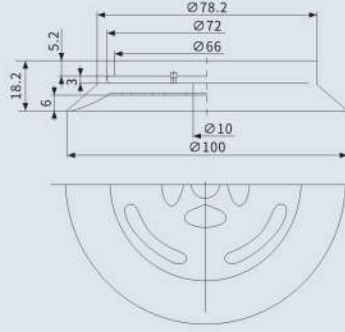
适合吸盘直径 Ø100
