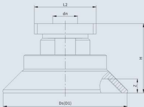
•MAF30~100RA(矩形适配器)
